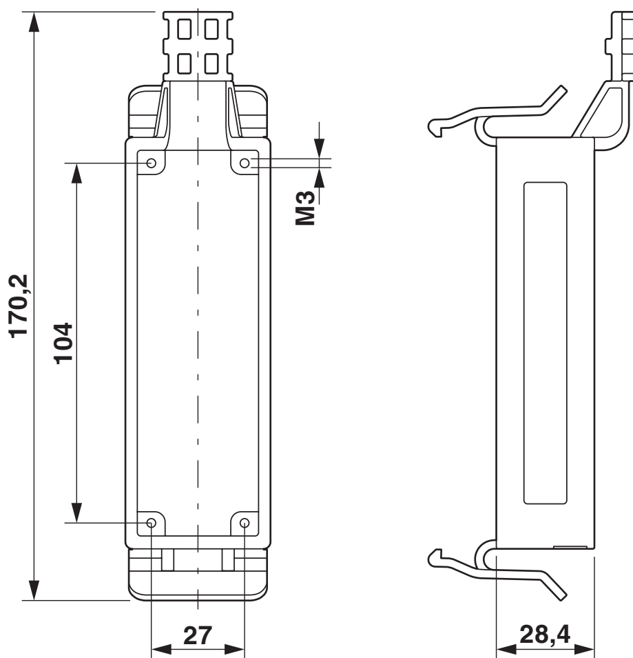
Dessin coté
