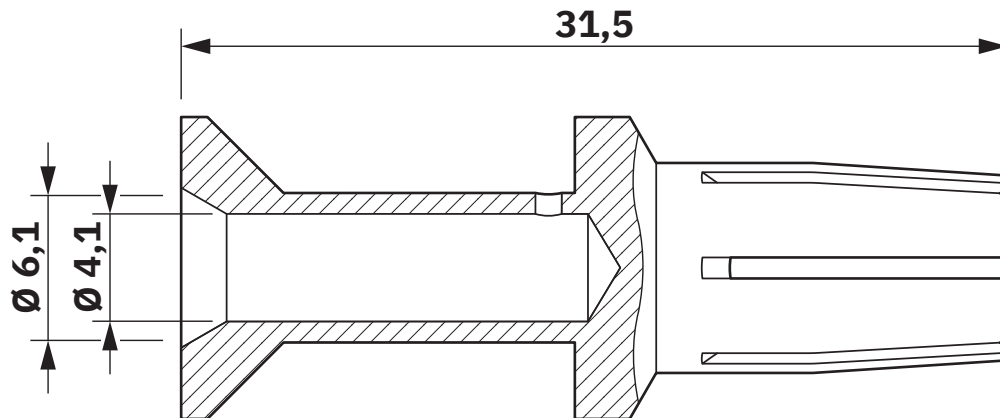
Dessin coté
