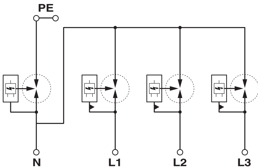
Schaltplan
