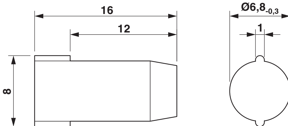
Maßzeichnung
