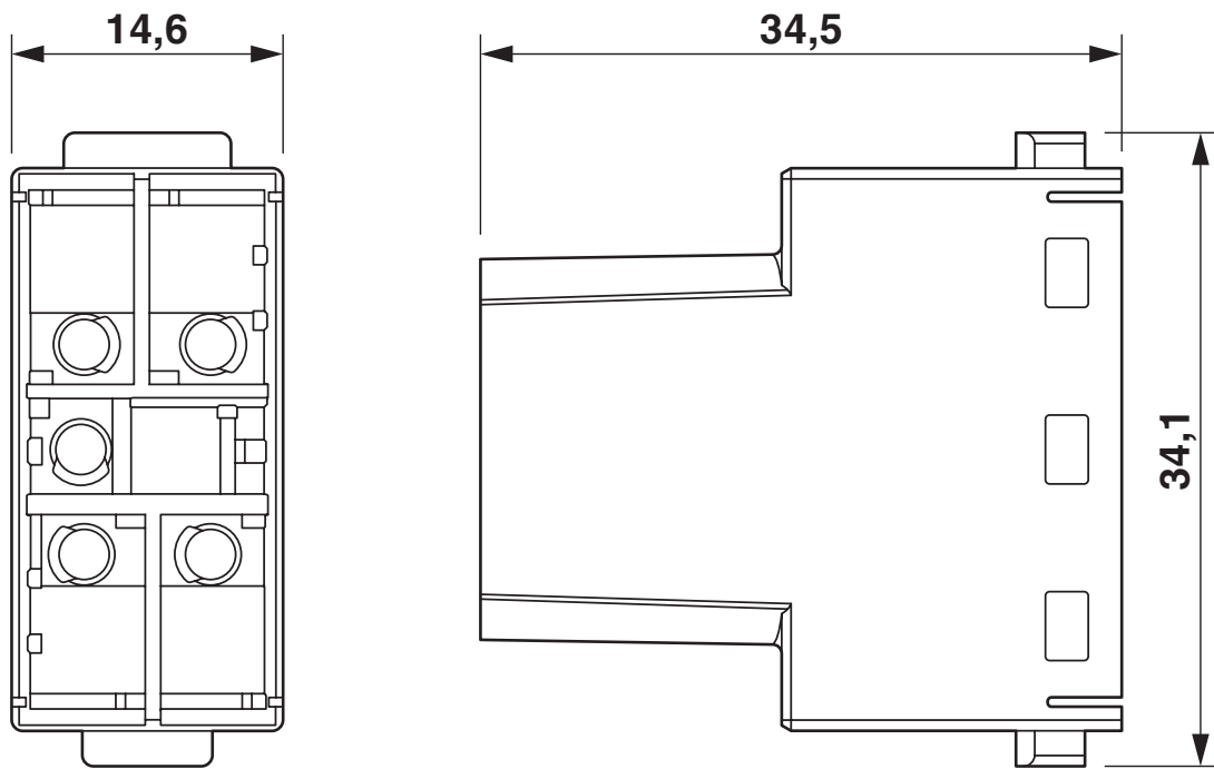
Maßzeichnung
