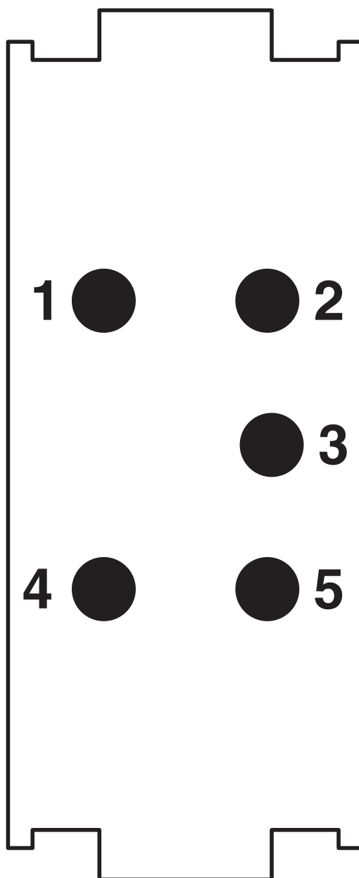
Schemazeichnung
