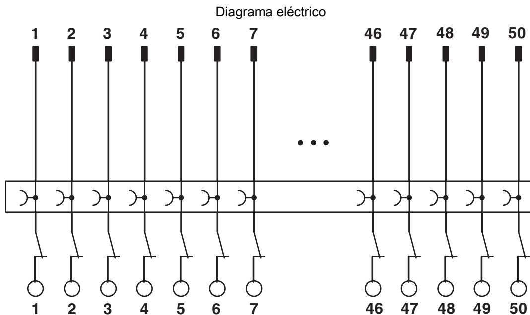
Esquema de conexiones FLKM 50/KDS3-MT/PPA/AN/PLC
