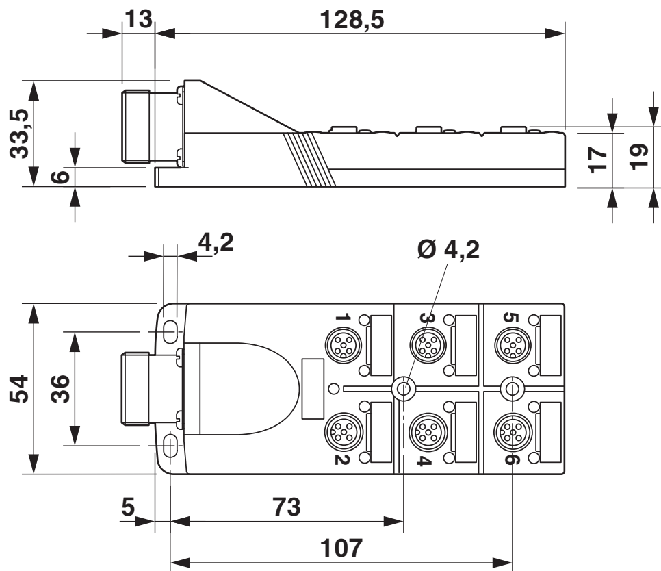
Dessin coté
