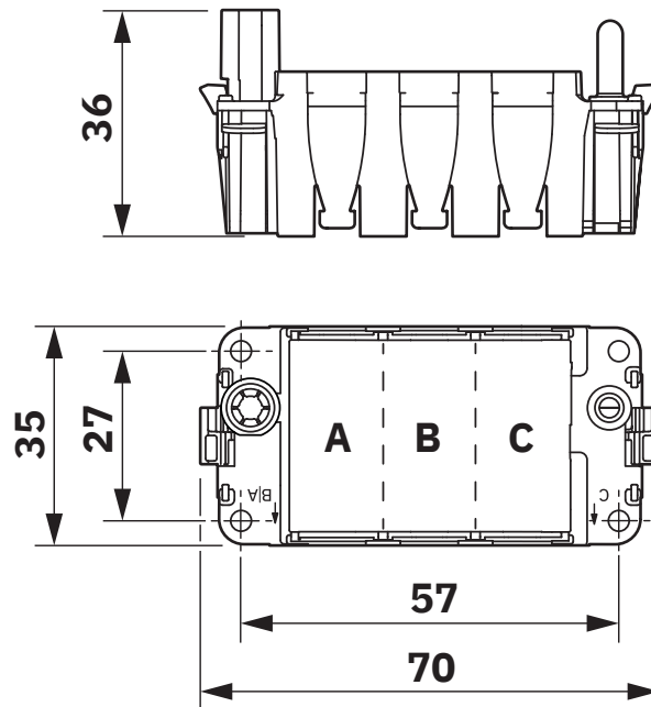
Maßzeichnung
