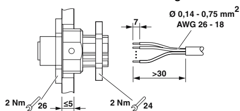
Funktionszeichnung
