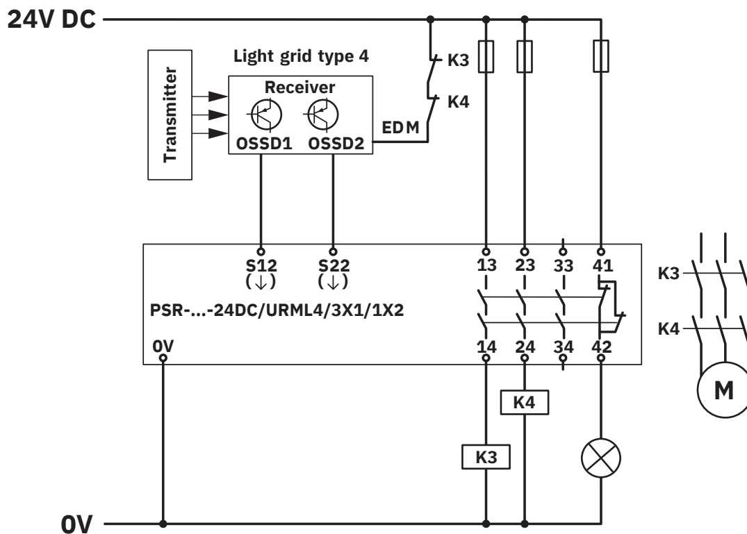
Zweikanalige Lichtgitterüberwachung
