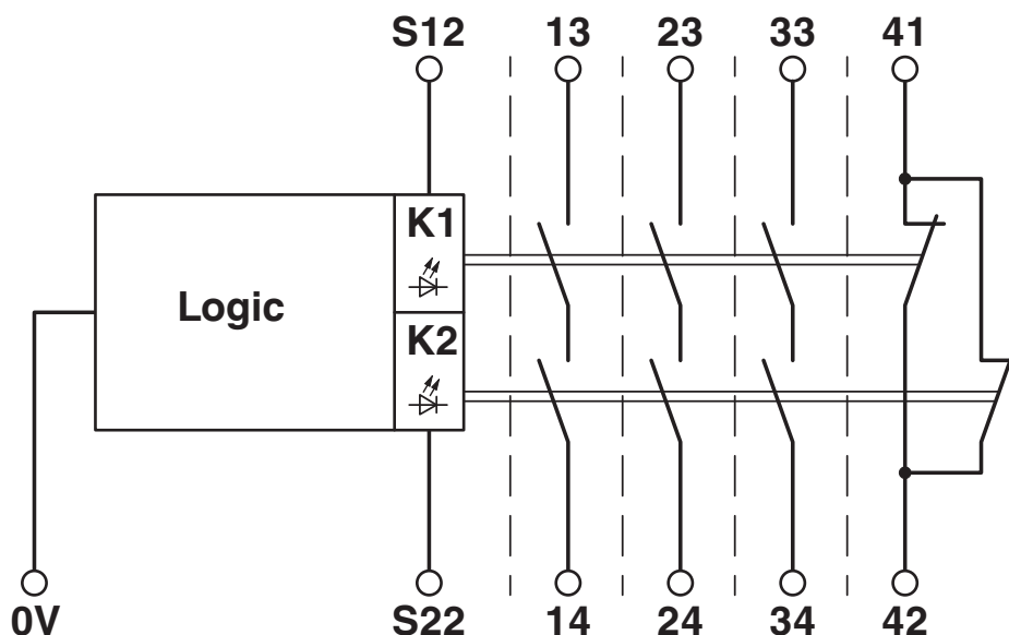
Schaltplan
