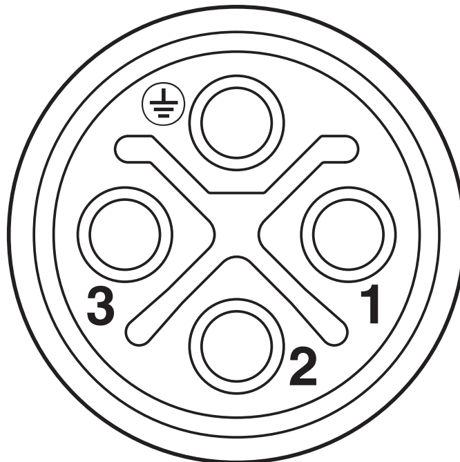
Schemazeichnung
