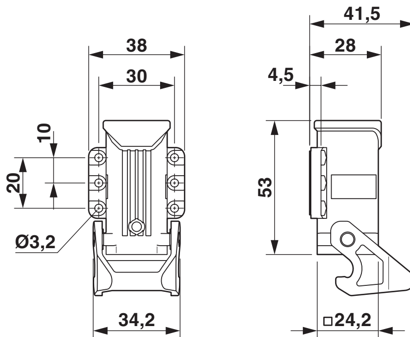
Dessin coté
