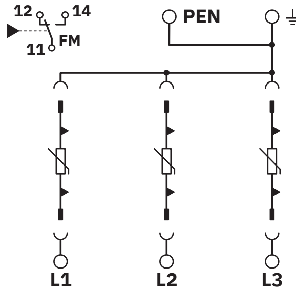
Diagrama eléctrico
