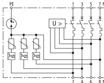
Prinzipschaltbild SPD+POP 4 255 C25
