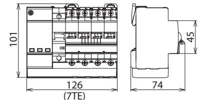
Maßbild SPD+POP 4 255 C25
