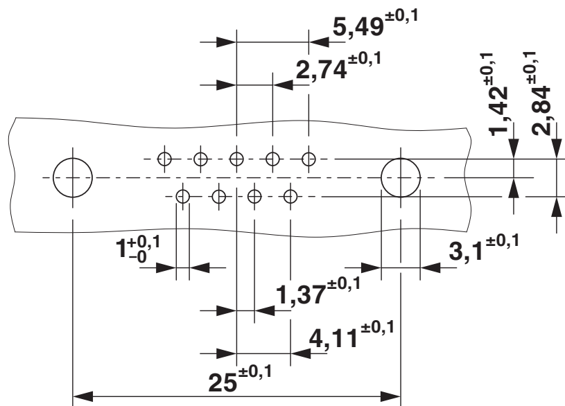
Bohrplan/Lötpadgeometrie
