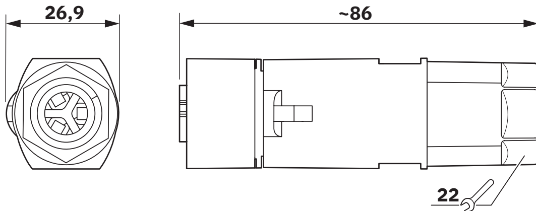
Maßzeichnung
