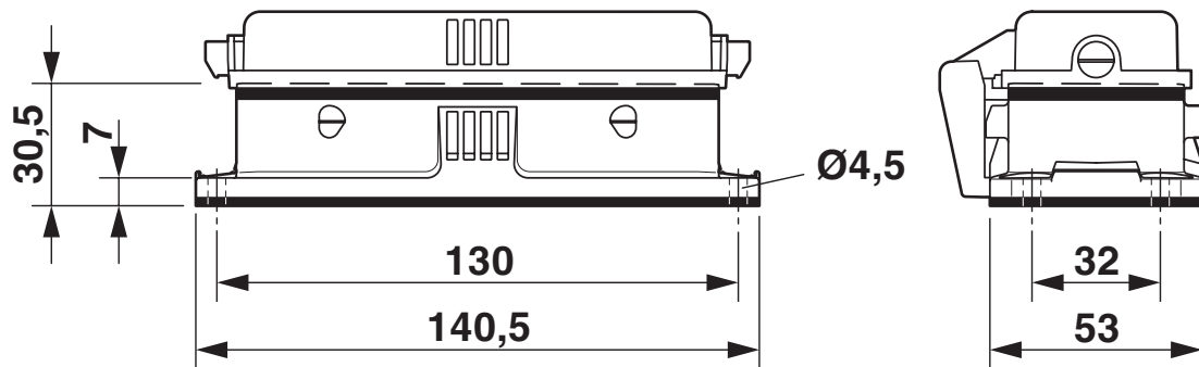
Maßzeichnung
