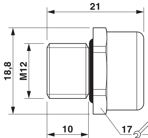
Maßzeichnung
