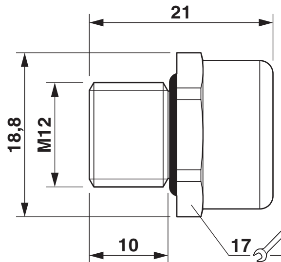
Dessin coté
