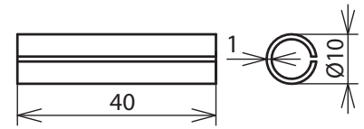
Maßbild CUPAH GL Q50 L40 CU AL
