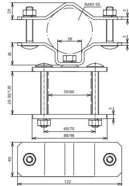
Maßbild BS D40.50 4K20.50 V2A
