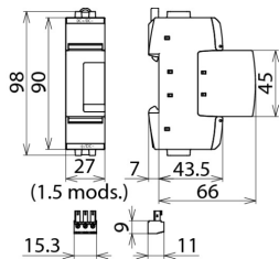
Dimensiones del DG SE DC 60 FM
