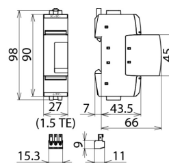
Dimensioni DG SE DC 60 FM
