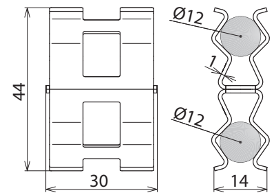
Maßbild DC BK 12 RD12 STBLANK
