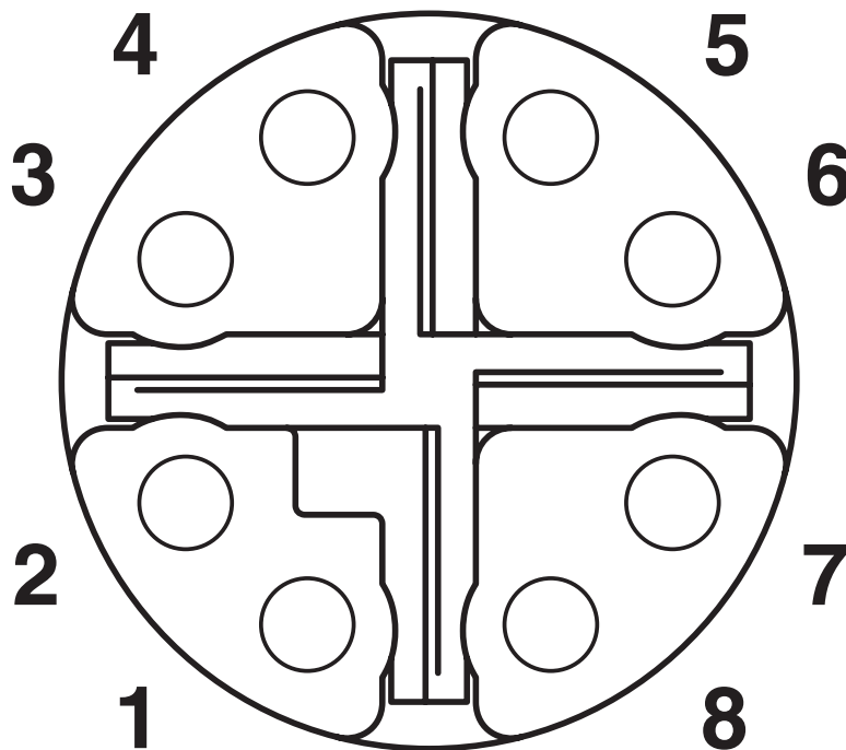
Plano esquemático
