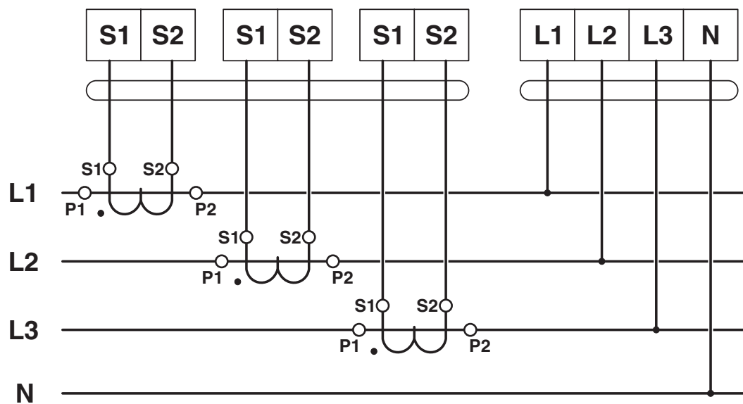
Diagrama eléctrico
