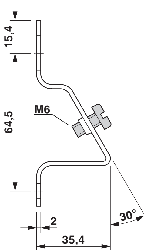
Dessin coté
