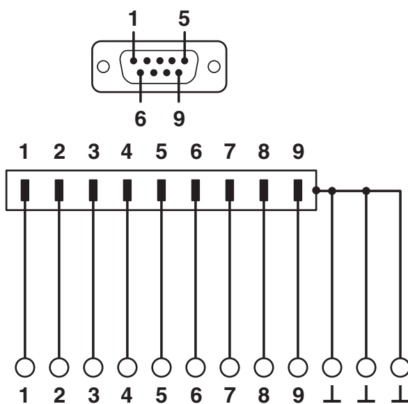
Schaltplan
