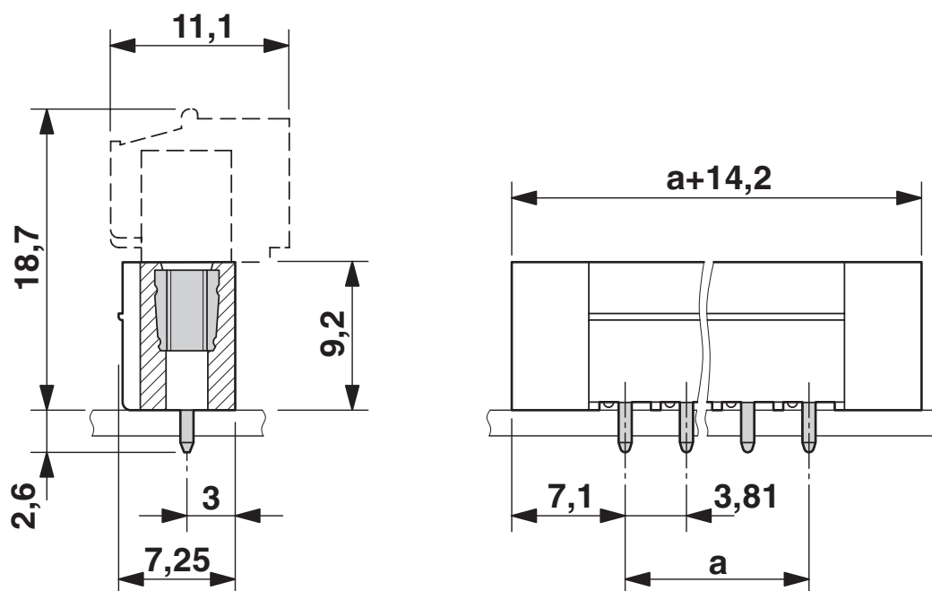
Dessin coté
