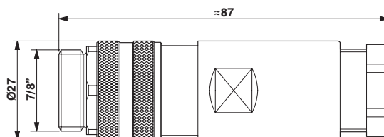
Maßzeichnung
