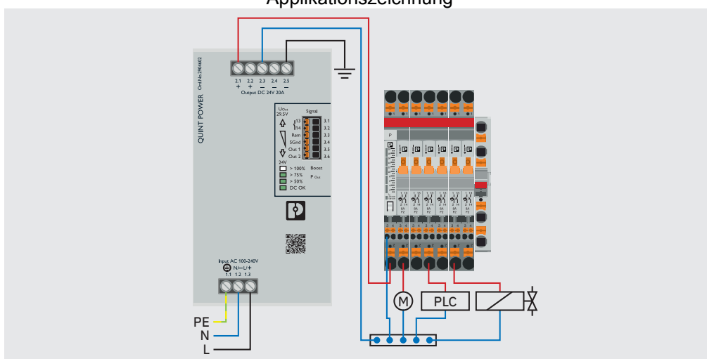
Applikationszeichnung
