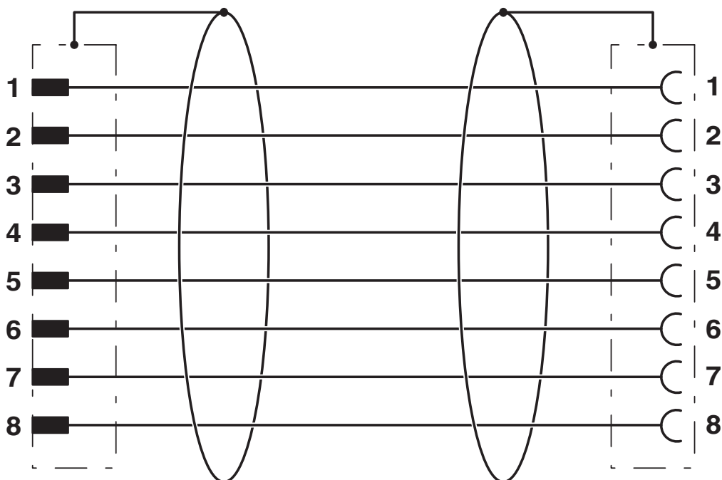
Schaltplan
