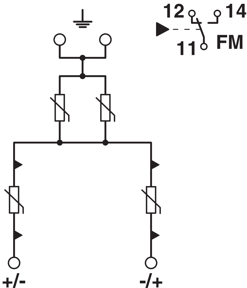
Schaltplan
