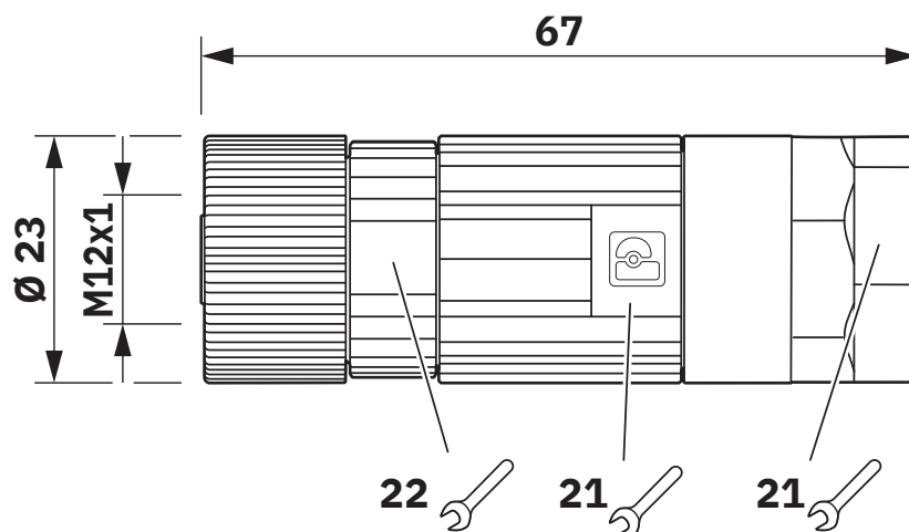
Maßzeichnung
