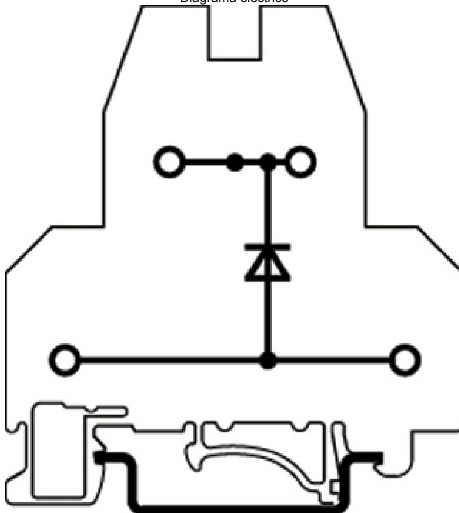
Diagrama eléctrico
