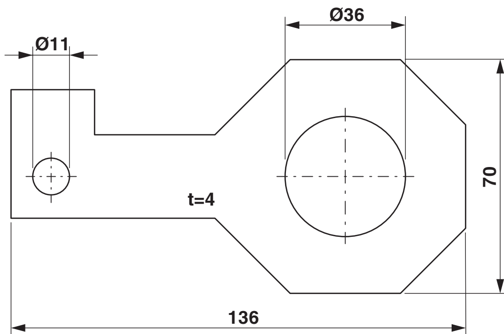
Dessin coté
