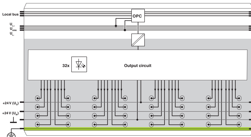
Schéma fonctionnel
