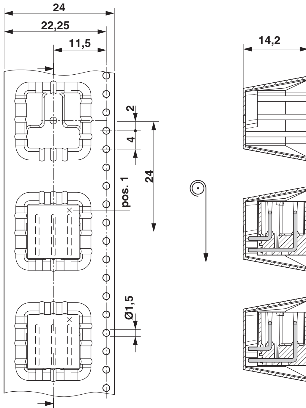
Maßzeichnung
