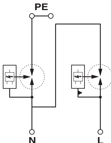
Diagrama eléctrico
