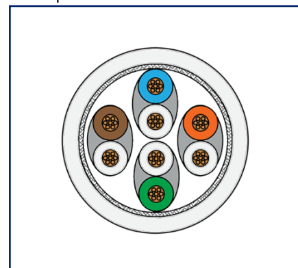
Prinzipbild
