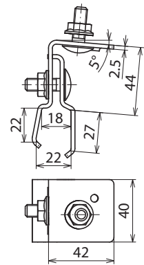
Maßbild HA M8 KF18.22 V2A
