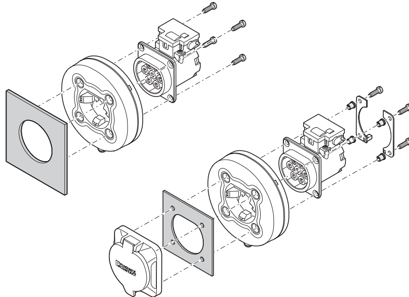
Explosionszeichnung
