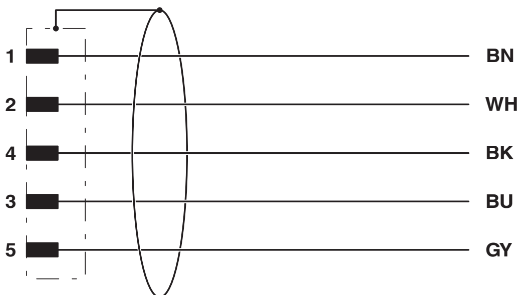
Diagrama eléctrico
