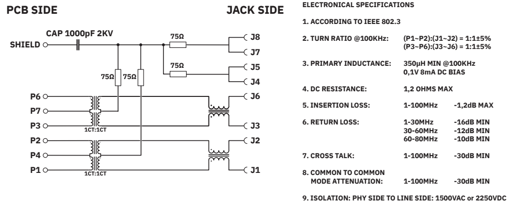
Diagrama eléctrico
