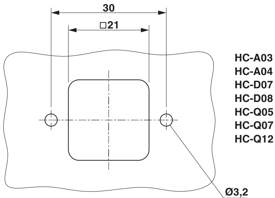
Maßzeichnung
