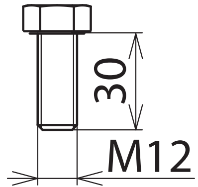
Maßbild SKS M12X30 V2A
