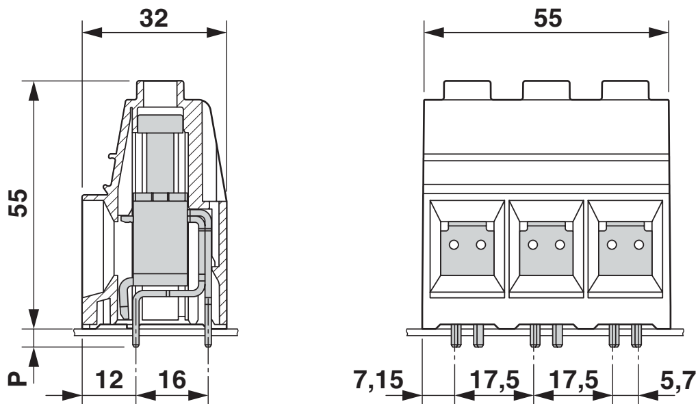
Dessin coté
