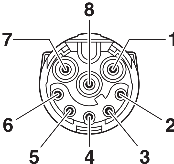
Plano esquemático
