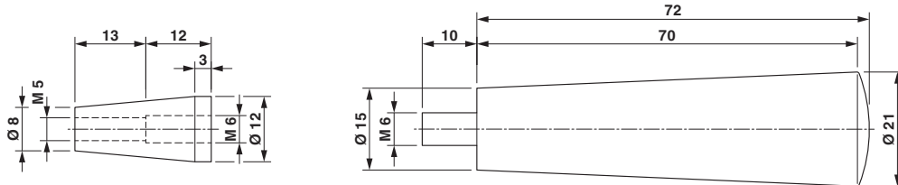
Maßzeichnung
