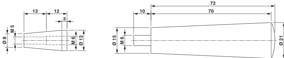
Esquema de dimensiones
